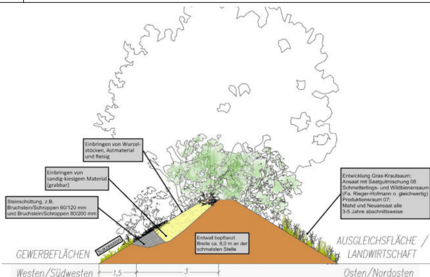
Schnitt durch das geplante Reptilienhabitat im Bereich des Walls
