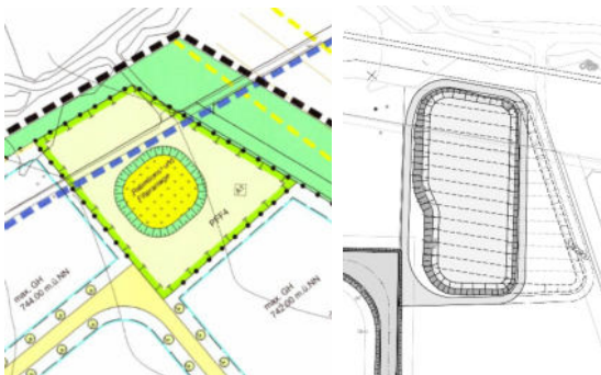
Abb. 1.4-4: Gegenüberstellung BPlan-Entwurf 2021 und aktuelle Erschließungsplanung Retention Nord
