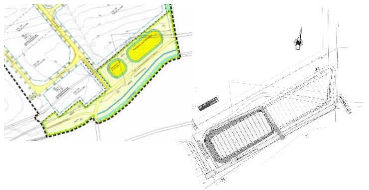
Abb. 1.4-5: Gegenüberstellung BPlan-Entwurf 2021 und aktuelle Erschließungsplanung Retention Süd
