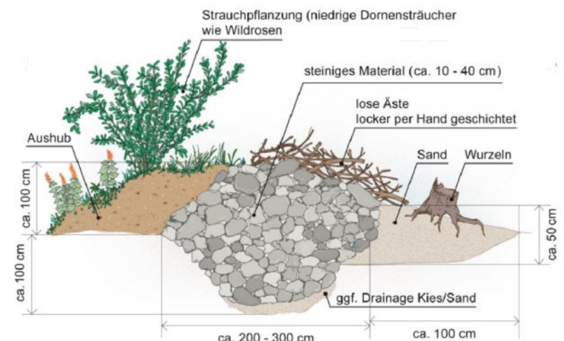
Querschnitt durch das geplante Reptilienhabitat (Grundlage / Quelle: Bayerisches Landesamt für Umwelt 2020)
